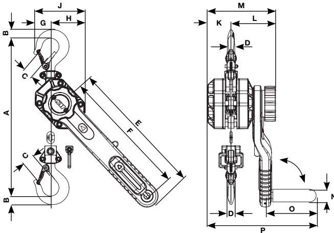
9 TON UNITS
